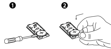
Figura 9: Inserção e remoção da bateria
